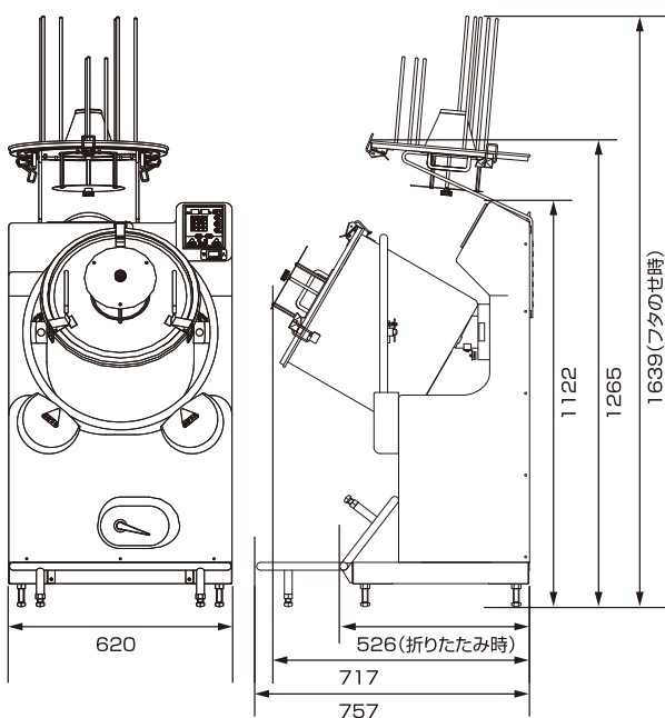
外観図 シャリロボ KS726B
